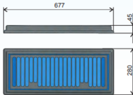
Filtro presa aria Filtre prise d'air Air intake filter Filter für Lufteingang Filtro por toma de aire
