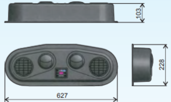
Diffusore aria Diffuseur d'air Air diffuser Luftverteiler Difusor aire
